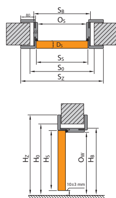
■ OŚCIEŻNICA PORTA SYSTEM ELEGANCE
