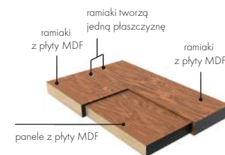
PRZEKRÓJ SKRZYDŁA LOGGIA PEŁNE
