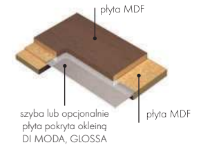
PRZEKRÓJ SKRZYDŁA BOLZANO
