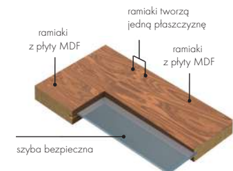
PRZEKRÓJ SKRZYDŁA LOGGIA Z PRZESZKLIENIEM
